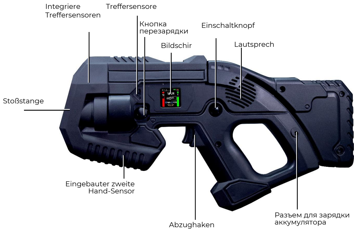
Die Hauptelemente des Tagers FALCON LUX (komplettiert als Premium)
