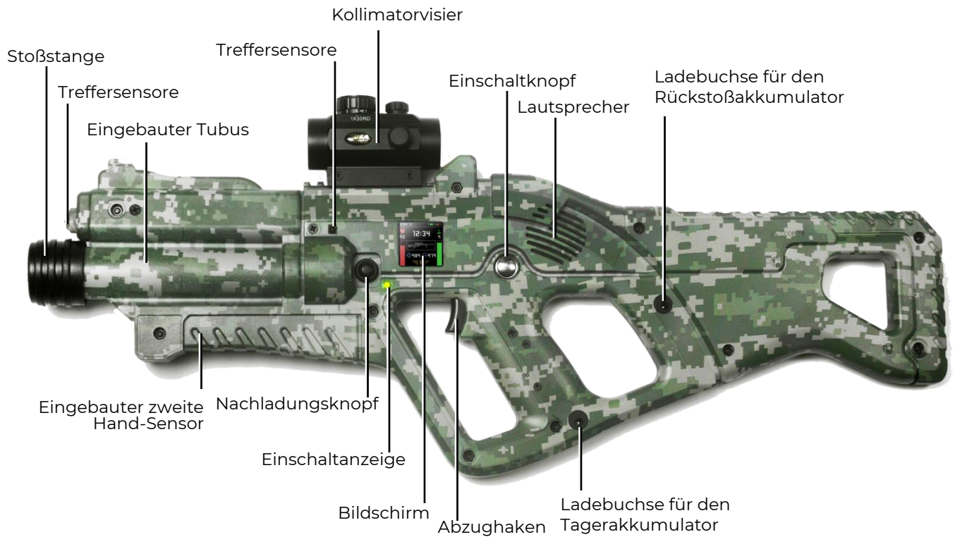
Die Hauptelemente des Tagers anhand der Sturmgewähr Falcon F2 (komplettiert als Tactical Pro)
